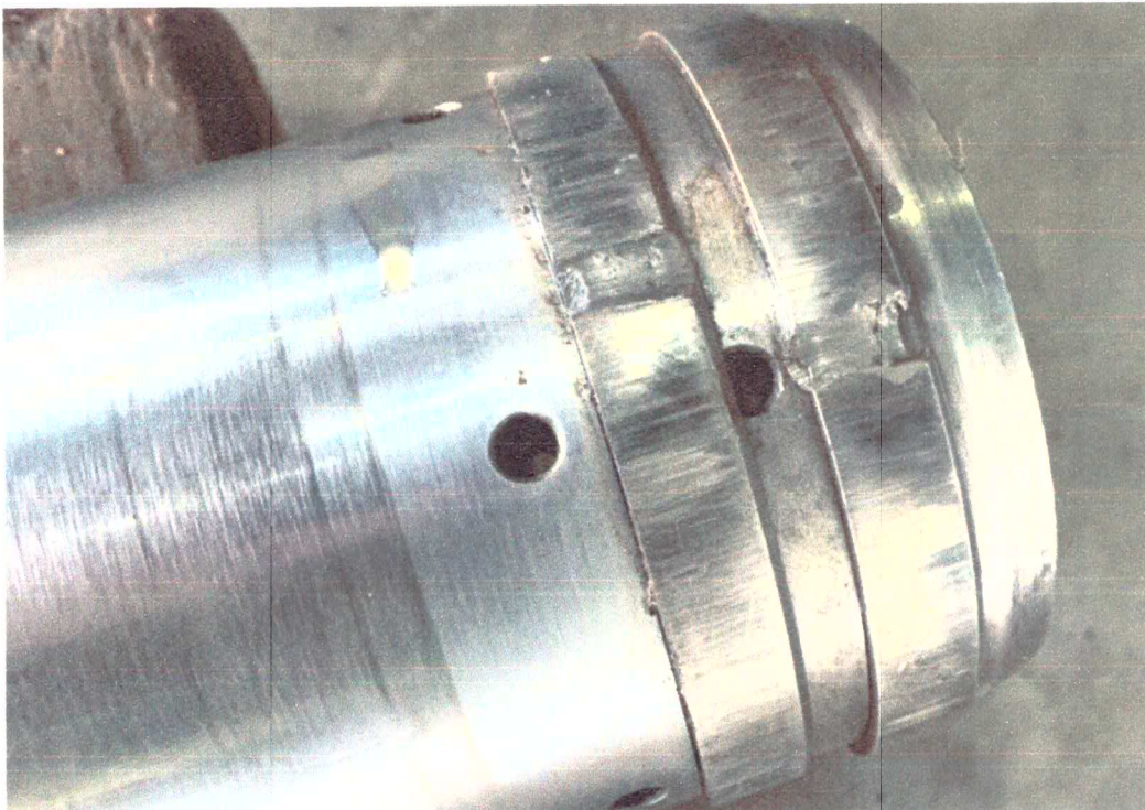
(parte desgastada onde gerou a limalha para danos no interior do cilindro)
