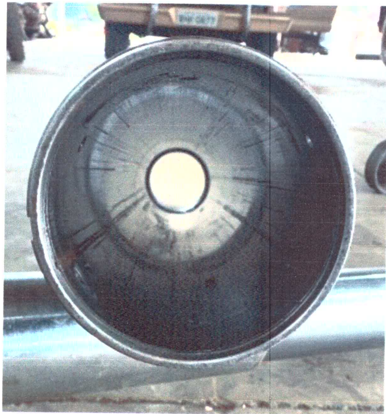
(parte interna cilindro onde gerava atrito e riscou a peça)
