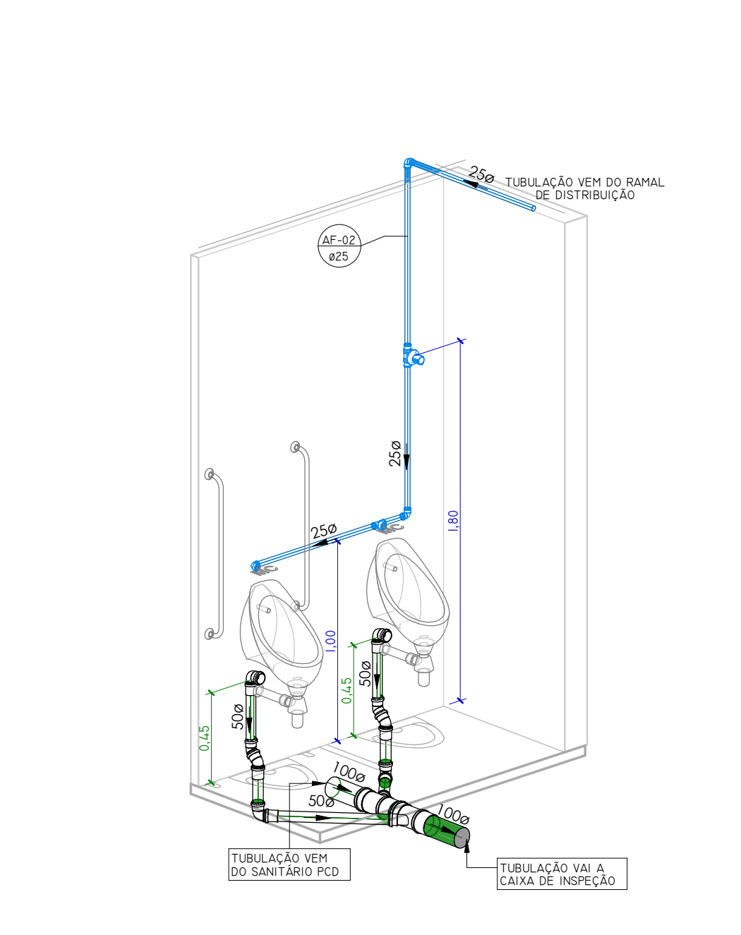
DETALHAMENTO MICTÓRIO SANITÁRIO MASCULINO
