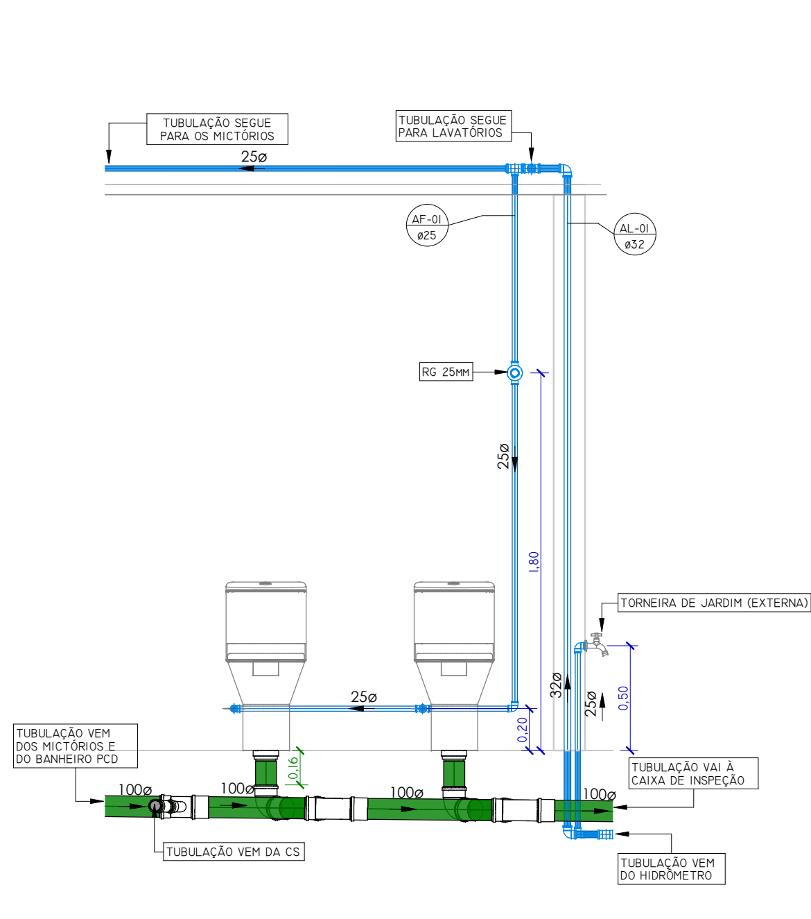
VISTA FRONTAL BACIA SANITÁRIA MASCULINO ESCALA 1 : 25
