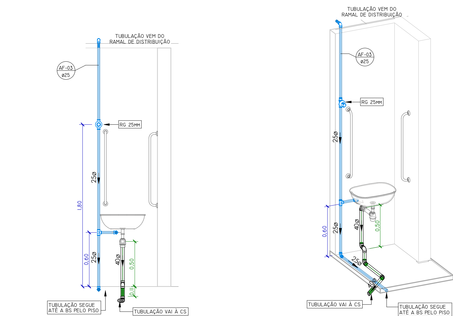
VISTA FRONTAL LAVATÓRIO PCD ESCALA 1 : 25
