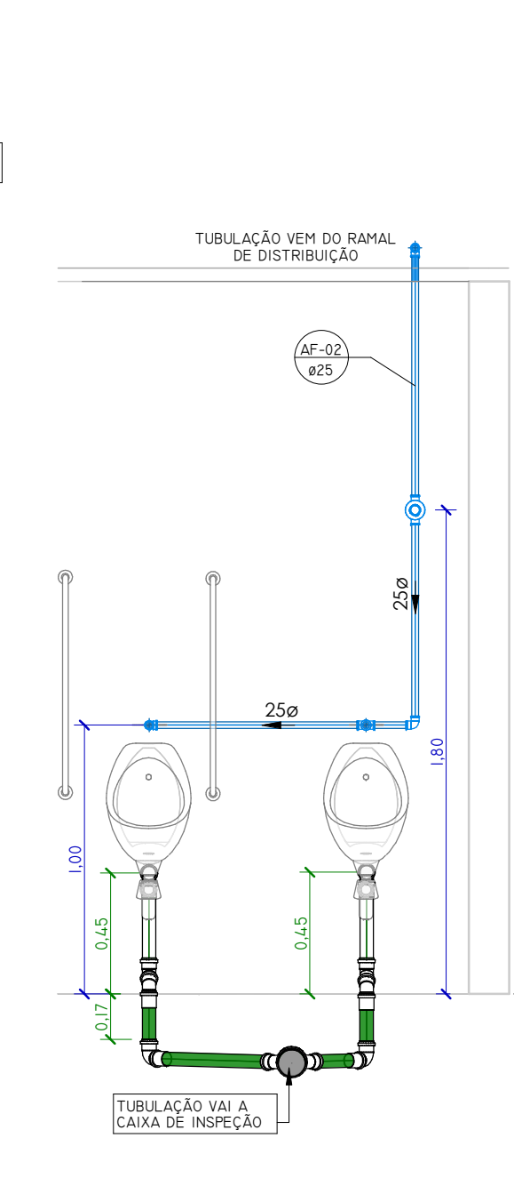
VISTA FRONTAL MICTÓRIO MASCULINO ESCALA 1 : 25
