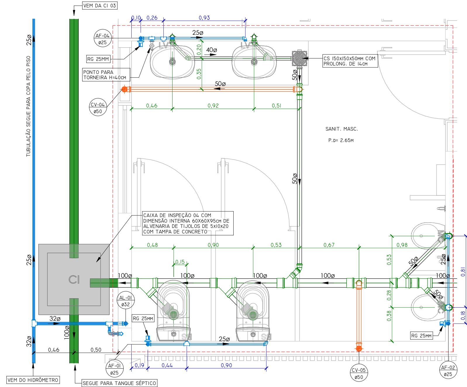
PLANTA BAIXA SANITÁRIO MASCULINO ESCALA 1 : 25
