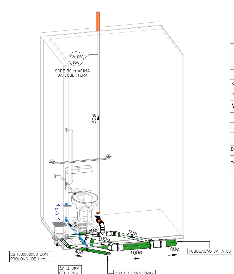
DETALHAMENTO BACIA SANITÁRIA PCD
