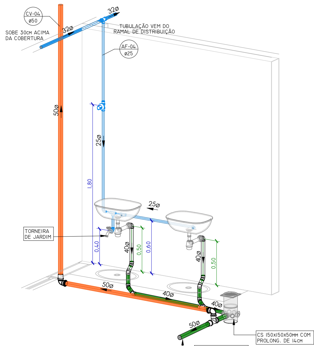
DETALHAMENTO LAVATÓRIO MASCULINO
