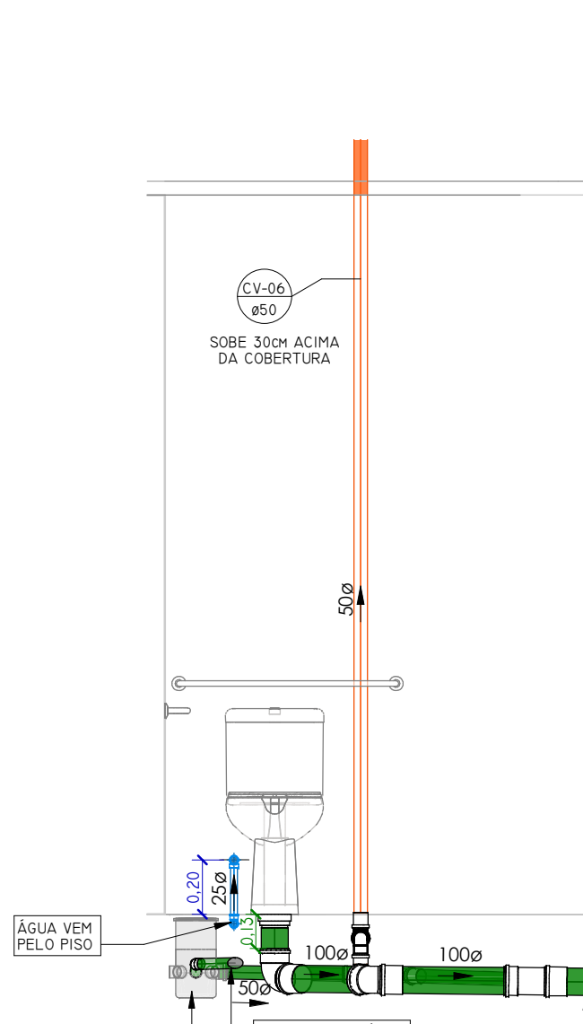
VISTA FRONTAL BACIA SANITÁRIA PCD ESCALA 1 : 25
