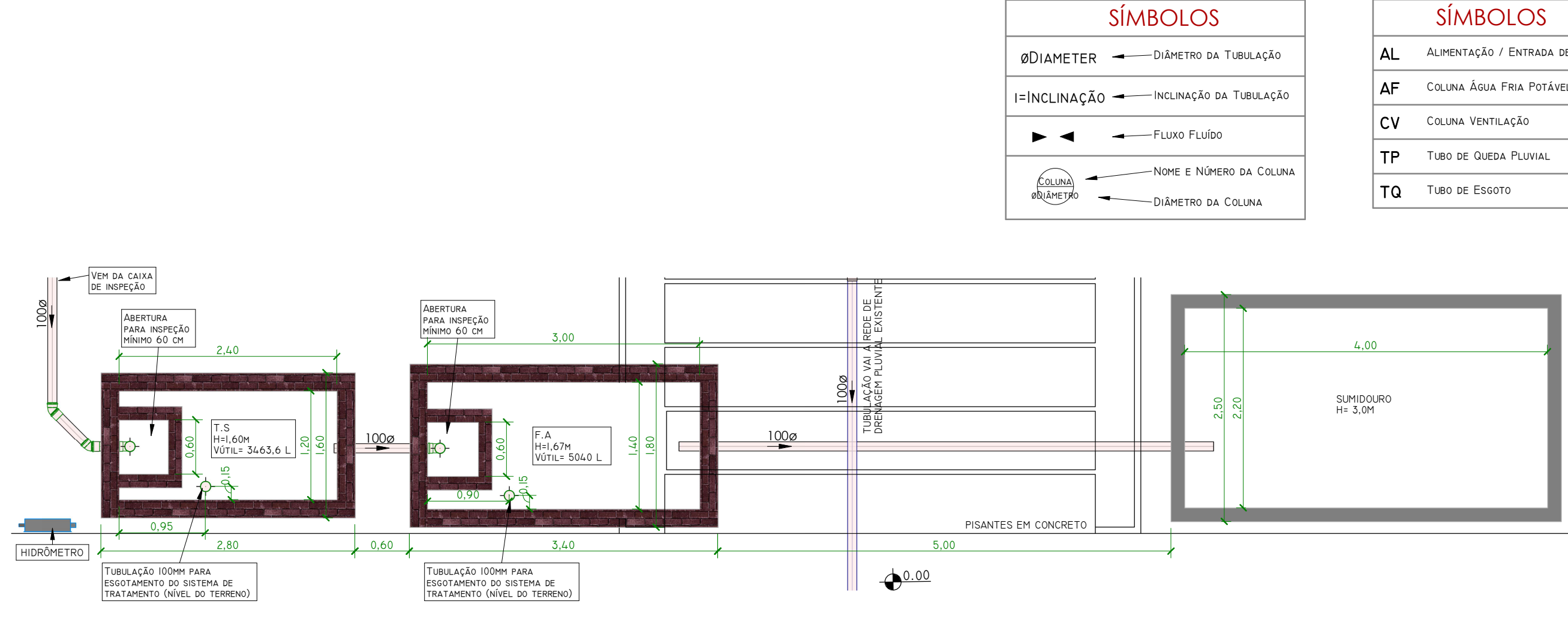
PLANTA BAIXA - TRATAMENTO DE ESGOTO ESCALA 1 : 50
