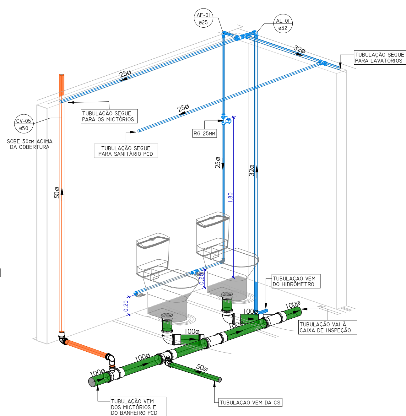
DETALHAMENTO BACIA SANITÁRIA MASCULINO
