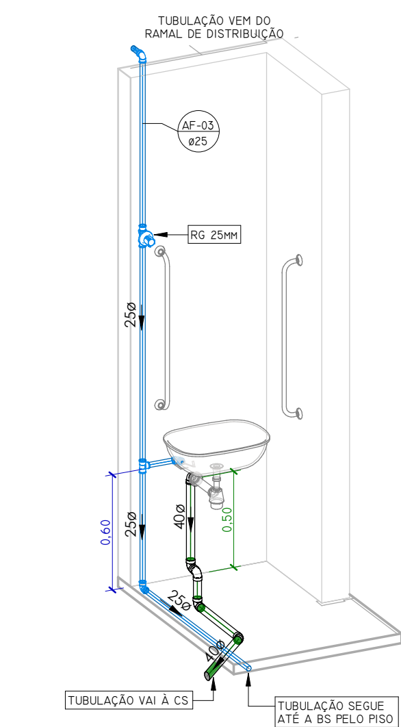
DETALHAMENTO LAVATÓRIO PCD
