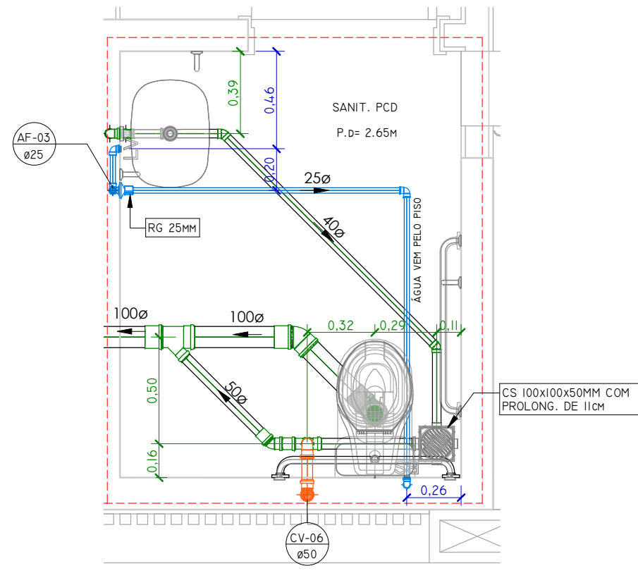
PLANTA BAIXA SANITÁRIO PCD ESCALA 1 : 25
