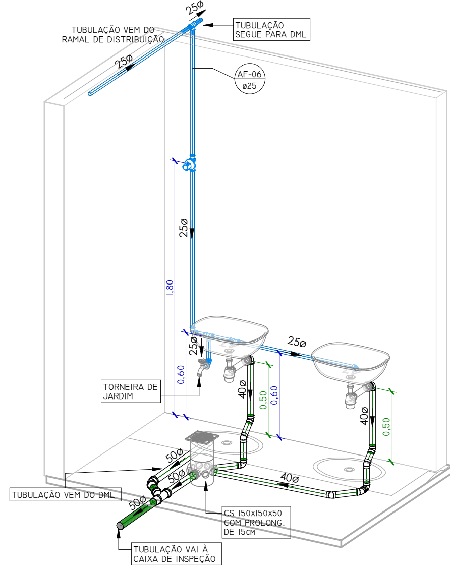
DETALHAMENTO LAVATÓRIO FEMININO
