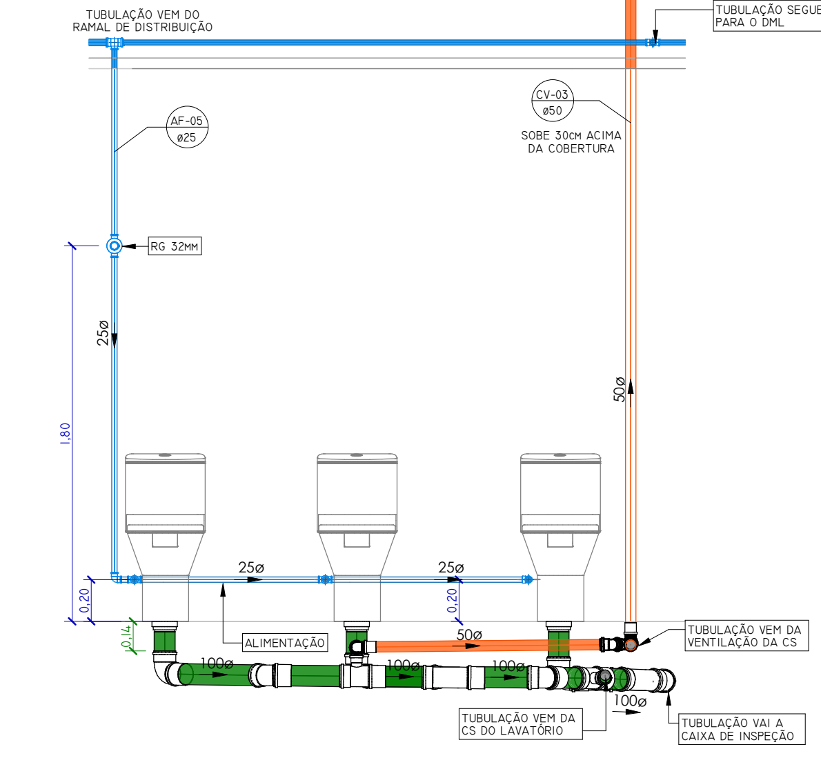
VISTA FRONTAL BACIA SANITÁRIA FEMININA
