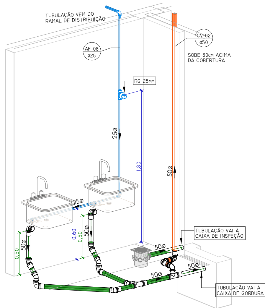
DETALHAMENTO COZINHA
