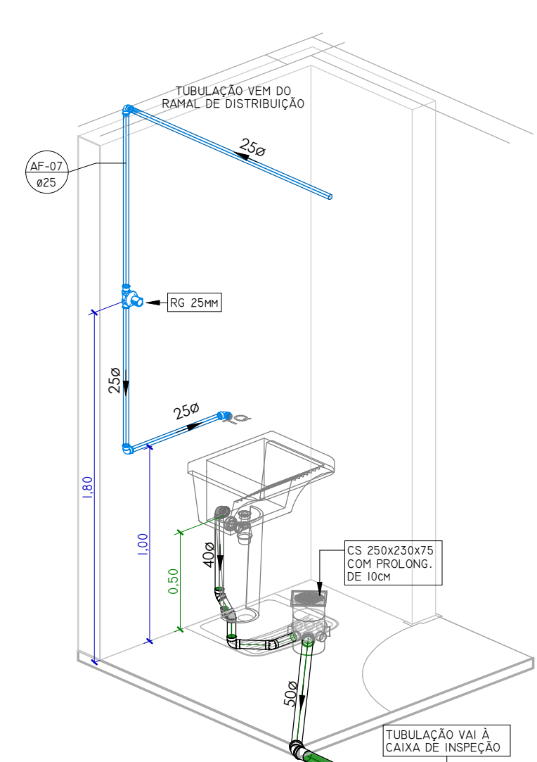
DETALHAMENTO DML
