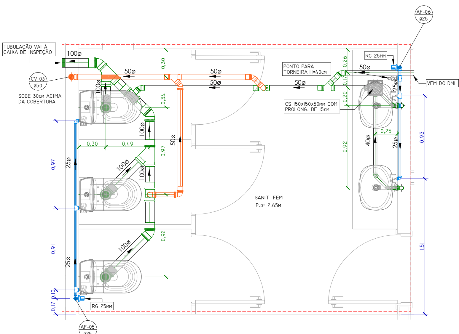
PLANTA BAIXA SANITÁRIO FEMININO
