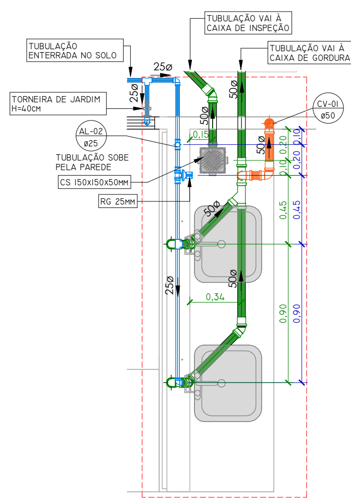
PLANTA BAIXA COPA
