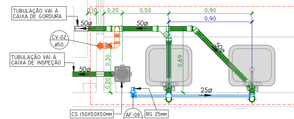
PLANTA BAIXA COZINHA
