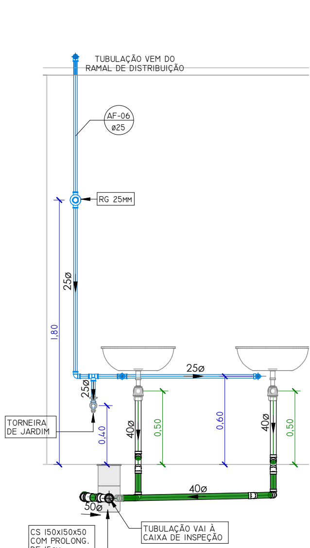
VISTA FRONTAL LAVATÓRIO FEMININO
