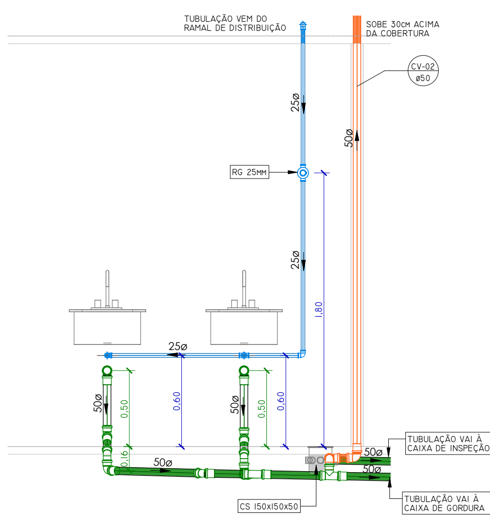
VISTA FRONTAL COZINHA
