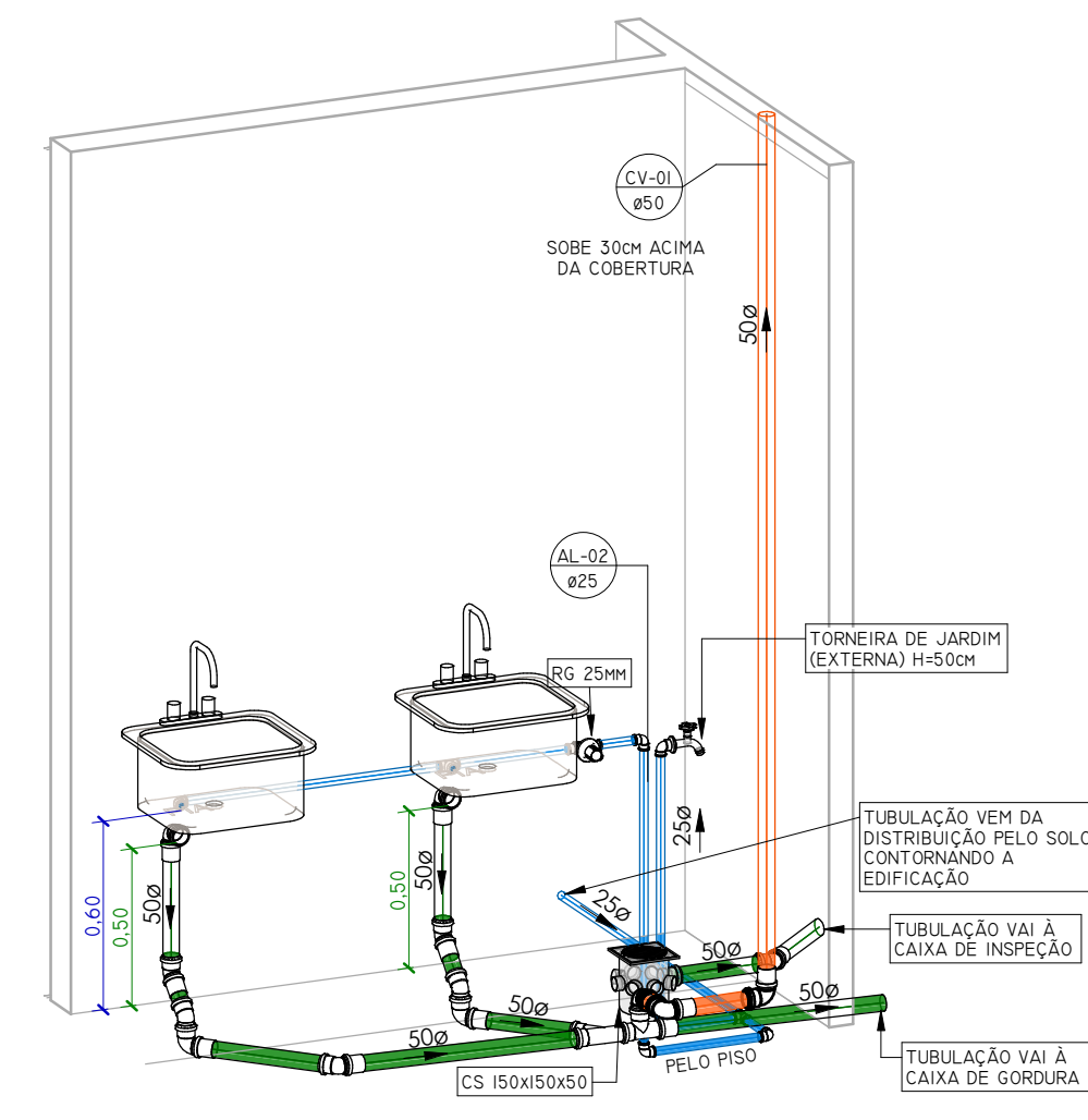
DETALHAMENTO COPA
