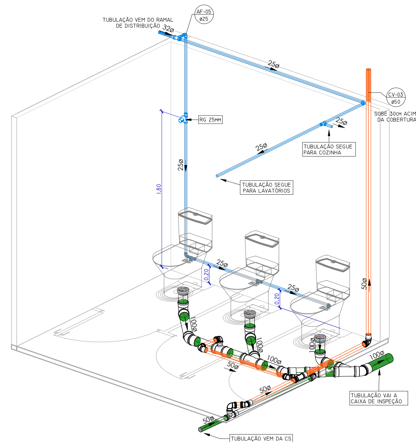
DETALHAMENTO BACIA SANITÁRIA FEMININA
