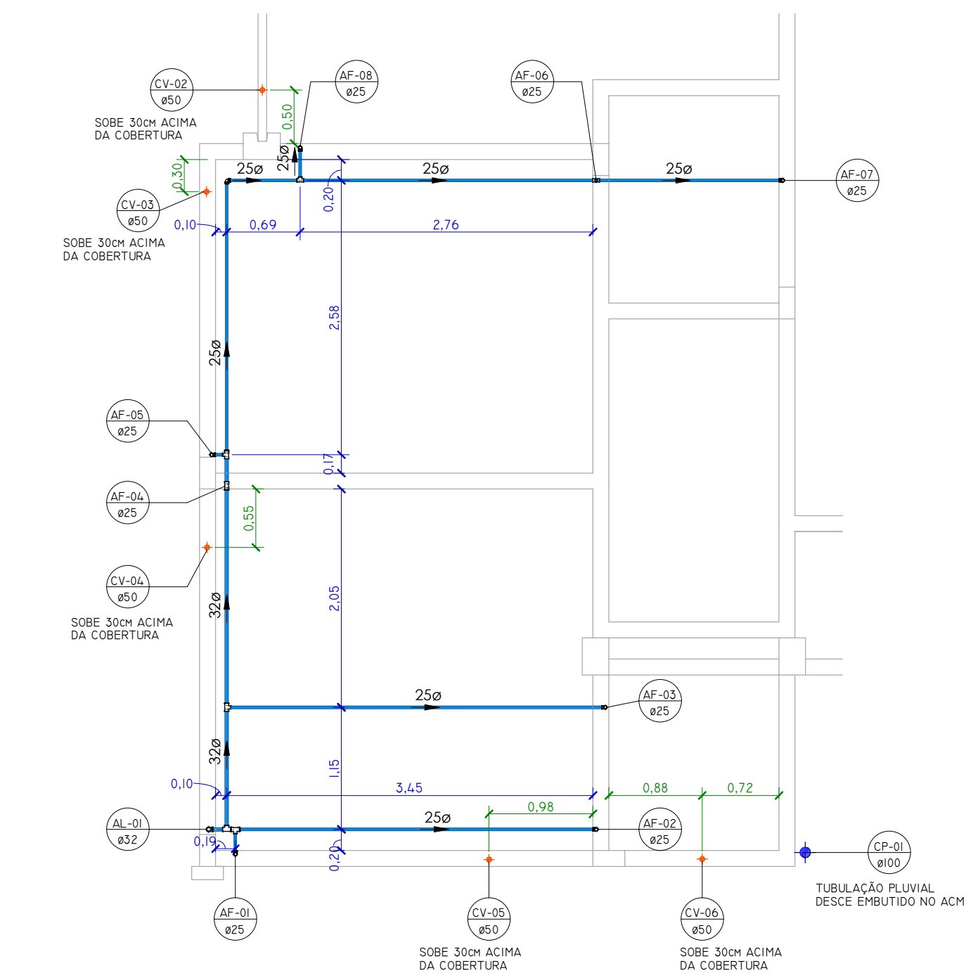
PLANTA BAIXA TUBULAÇÃO FORRO
