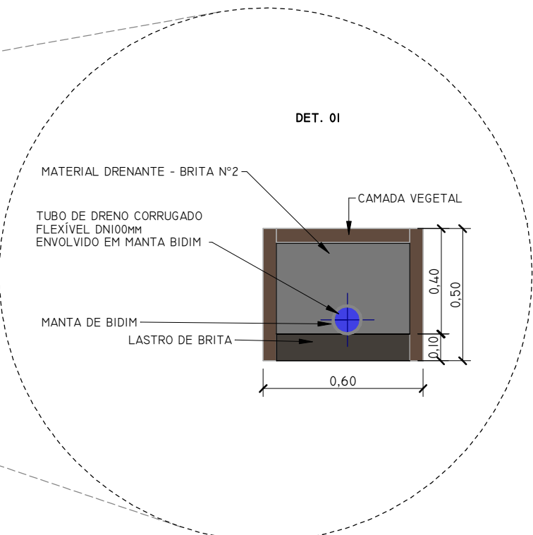
DETALHAMENTO TUBO DE DRENAGEM ESCALA 1 : 20
